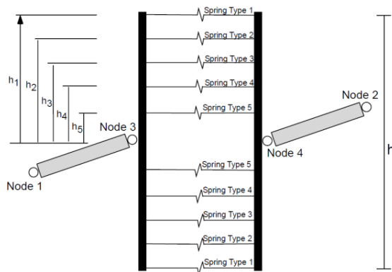
شکل ۲- اساس مدل‌سازی اتصال گهواره‌ای در روش چند فنی (۱۰ فز) [۱۲]
