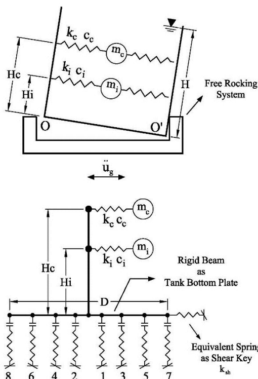
شکل ۴- (بالا) مدل مکانیکی و (پایین) شمای کلی مدل عددی سازه مخزن با امکان حرکت گهواره‌ای آزاد در نرم‌افزار OpenSees
