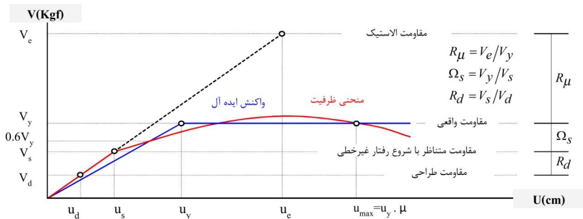
شکل ۱۳- دوحطی سازی منحنی ظرفیت سازه و معرفی پارامترهای مربوط به محاسبه ضریب رفتار
