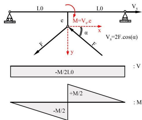
شکل ۴- نمودار آزاد تیر طبقه، تغییرات برش و لنگر خمشی در آن
