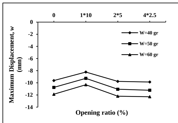
شکل ۱۷- رابطه‌ی تغییر مکان صفحه با درصد بازشوهای دایره‌ای با سطح یکسان و موقعیت قرارگیری متفاوت
