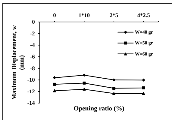
شکل ۱۸- رابطه‌ی تغییر مکان صفحه با درصد بازشوهای مربعی با سطح یکسان و موقعیت قرارگیری متفاوت
