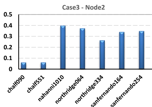
شکل ۱۳- جابجایی افقی در حالت تاریخیچه زمانی غیرخطی برای سازه یک طبقه
