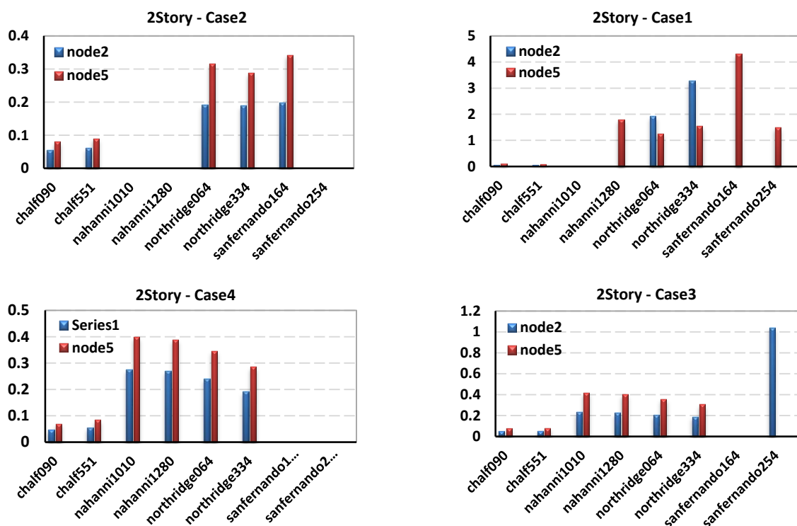
شکل ۱۴- جابه جایی در جهت x در حالت تاریخچه زمانی غیرخطی برای سازه ۲ طبقه
