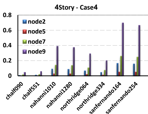
شکل ۱۲- جابجایی افقی در حالت تاریخیچه زمانی خطی برای سازه ۴ طبقه
