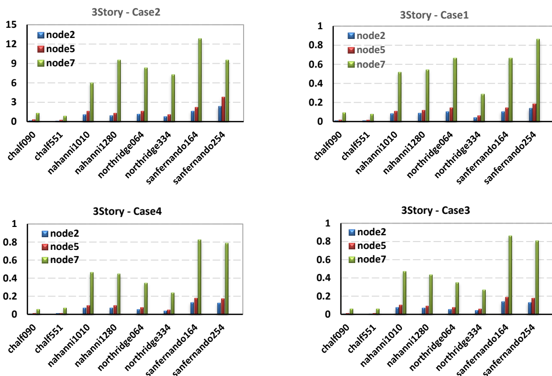
شکل ۱۱- جابجایی افقی در حالت تاریخیچه زمانی خطی برای سازه ۳ طبقه
