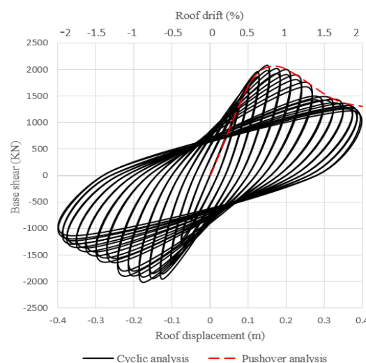
الف) تطابق منحنی هیستریزس حاصل از تحلیل چرخه‌ای و منحنی پوش حاصل از تحلیل استاتیکی غیرخطی افزایشده سیستم SMF&CSWs
