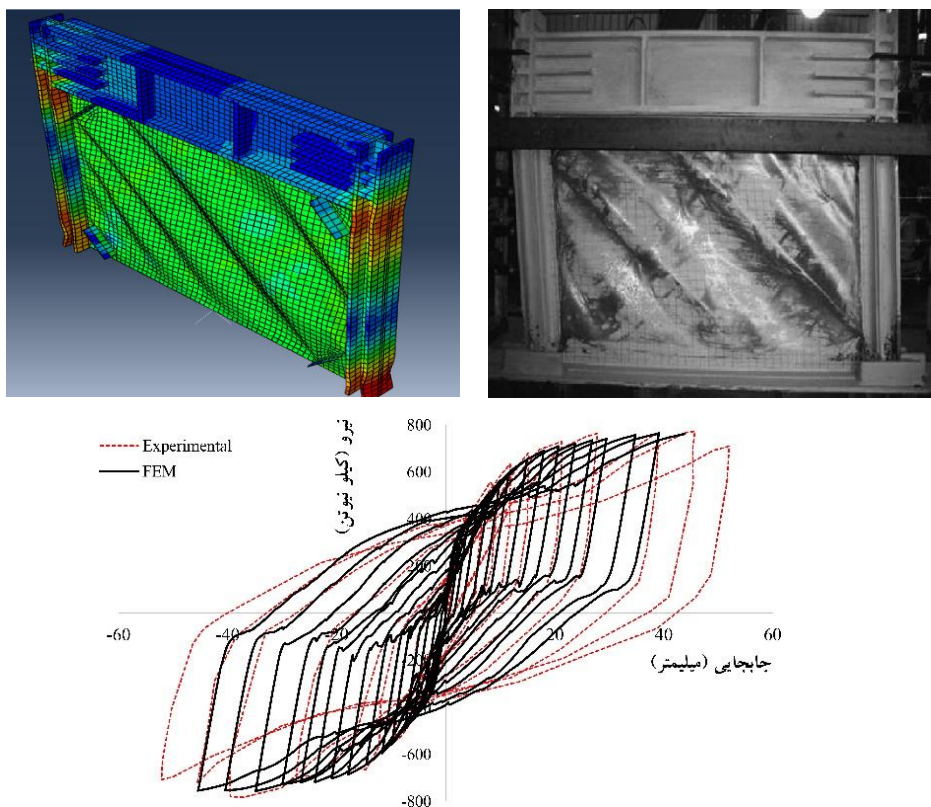
شکل ۷- اعتبار سنجی نتایج آزمایشگاهی با نتایج حاصل از شبیه‌سازی [۲۲]
