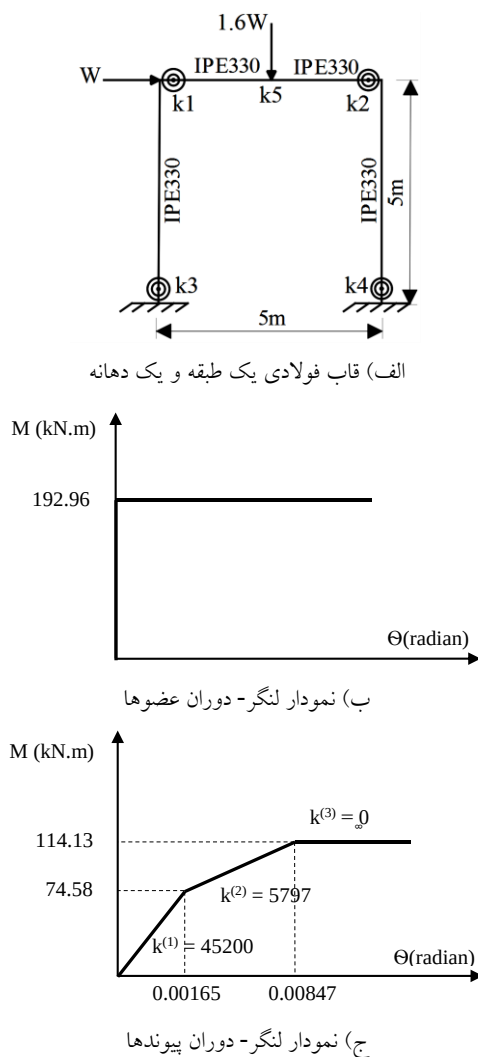
شکل ۱- قاب فولادی یک طبقه و یک دهانه و رفتار کشسان-مومسان عضوها و پیوندها [۱۸]
