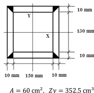
شکل ۴- مقطع ستون ساخته شده با جوش شیار با نفوذ کامل در نمونه شاهد آزمایش
