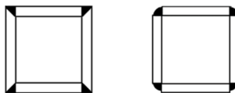
شکل ۲- مقطع جعبه‌ای ساخته‌شده از ورق با دو نوع جوش
