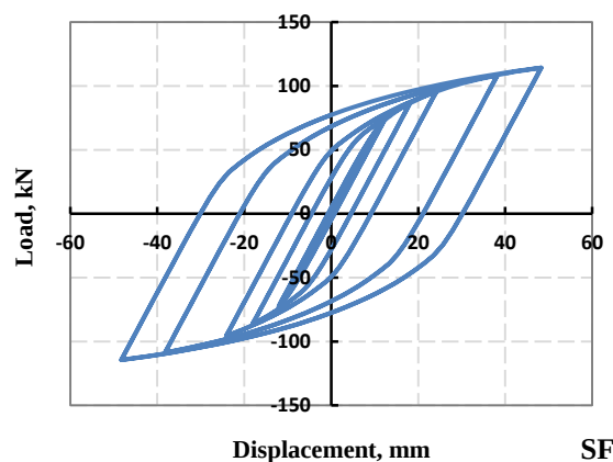
شکل ۱۱- منحنی نیرو-جابجایی (هیستریزیس) برای نمونه قاب خمشی ویژه با ستون جعبه‌ای ساخته شده با جوش گوشه (SF)
