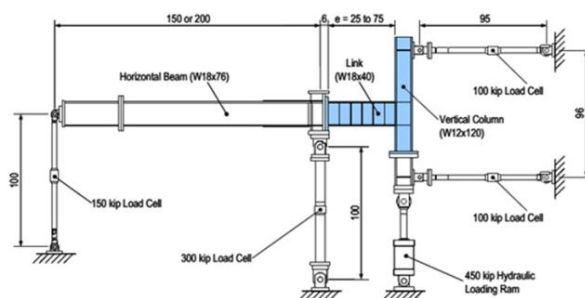
شکل ۵- ساختار مدل ایجاد شده در برنامه ABAQUS
