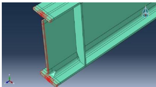
شکل ۲- جزئیات سوراخ دسترسی جوش
