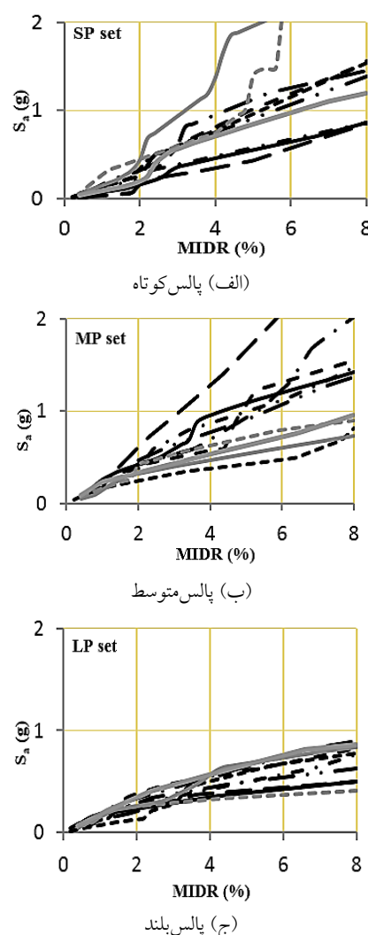
شکل ۳- منحنی‌های IDA قاب ۱۵ طبقه تحت مجموعه رکوردهای مورد مطالعه
