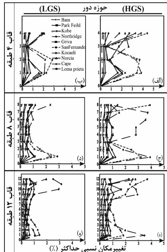
شکل ۶- تغییر مکان نسبی بین طبقاتی در قاب های مورد مطالعه برای زلزله حوزه دور تحت تحلیل های تاریخچه زمانی غیرخطی
