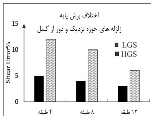
شکل ۱۴- اختلاف ناشی از رکوردهای نزدیک و دور از گسل در محاسبه برش پایه در سازه‌های مورد مطالعه
