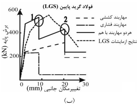
شکل ۴- تعریف مفاصل در مهاربندها با توجه به آزمایشات عبادی و صبور، (الف) HGS، (ب) LGS [۵]
