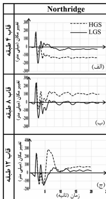
شکل ۱۰- مقایسه اثر تغییر مکان ماندگار (Fling Step)، برای مدل‌های طراحی شده با فولاد LGS و HGS تحت زلزله حوزه نزدیک نورتریج
