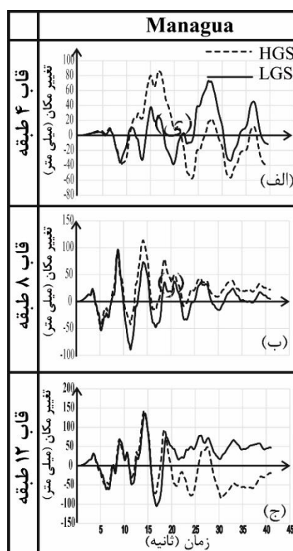
شکل ۱۱- مقایسه اثر تغییر مکان ماندگار (Fling Step)، برای مدل‌های طراحی شده با فولاد LGS و HGS تحت زلزله حوزه نزدیک ماناگوا
