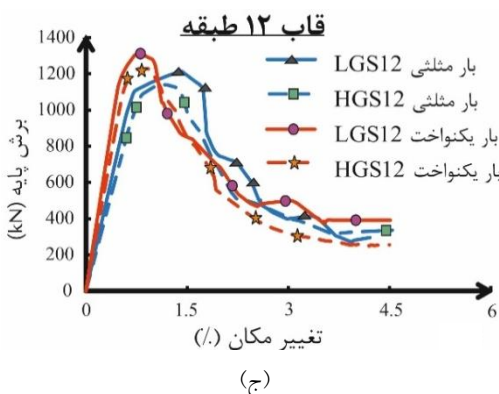
شکل ۳- منحنی‌های ظرفیت قالب‌ها، (الف) ۴ طبقه، (ب) ۸ طبقه و (ج) ۱۲ طبقه
