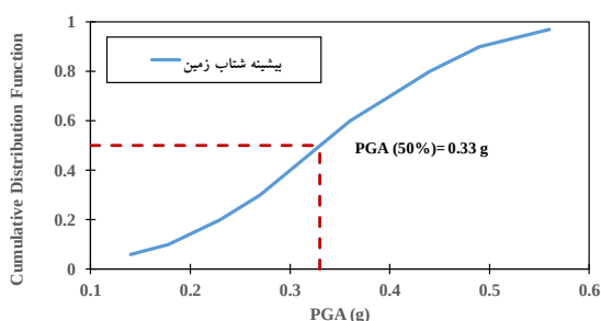
شکل ۲- منحنی CDF بر اساس تابع توزیع تجمعی نرمال برای پارامتر بیشینه شتاب زمین فهرست پیشنهادی
