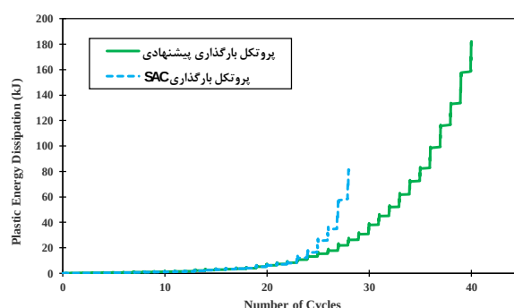
شکل ۱۸- انرژی پلاستیک مستهلک شده در نمونه‌های آزمایشگاهی WUF-W در مقادیر هدف پروتکل‌های بارگذاری ملی و SAC
