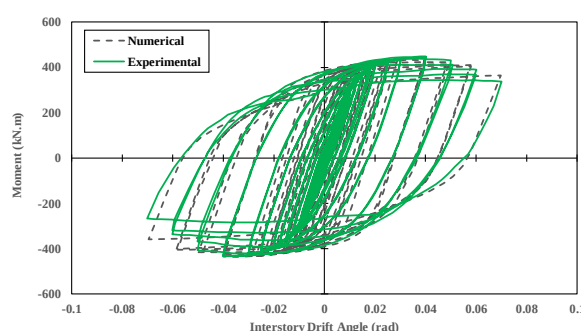
شکل ۲۶- منحنی رفتاری نمونه آزمایشگاهی و مدل عددی اتصال خمشی WUF-W تحت پروتکل بارگذاری ملی
