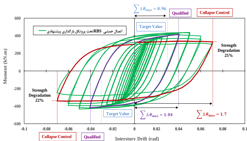
شکل ۱۹- منحنی رفتاری نمونه اول اتصال خمشی RBS تحت پروتکل بارگذاری ملی
