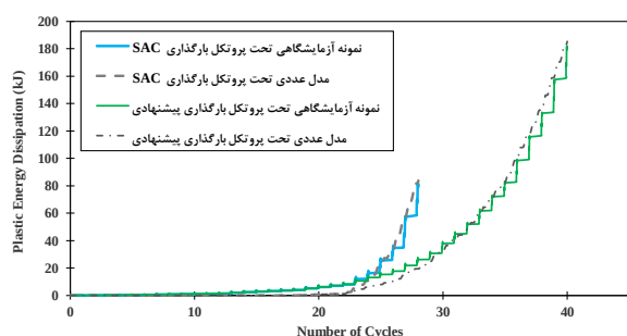
شکل ۲۷- مقایسه انرژی پلاستیک مستهلک شده در مدل عددی و نمونه‌های آزمایشگاهی اتصال WUF-W در شرایط پذیرش پروتکل‌های بارگذاری ملی و SAC
