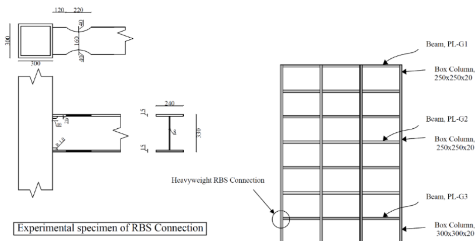
شکل ۹- جزئیات نمونه آزمایشگاهی اتصال RBS در قاب ۷ طبقه (ابعاد بر حسب سانتی متر هستند).
