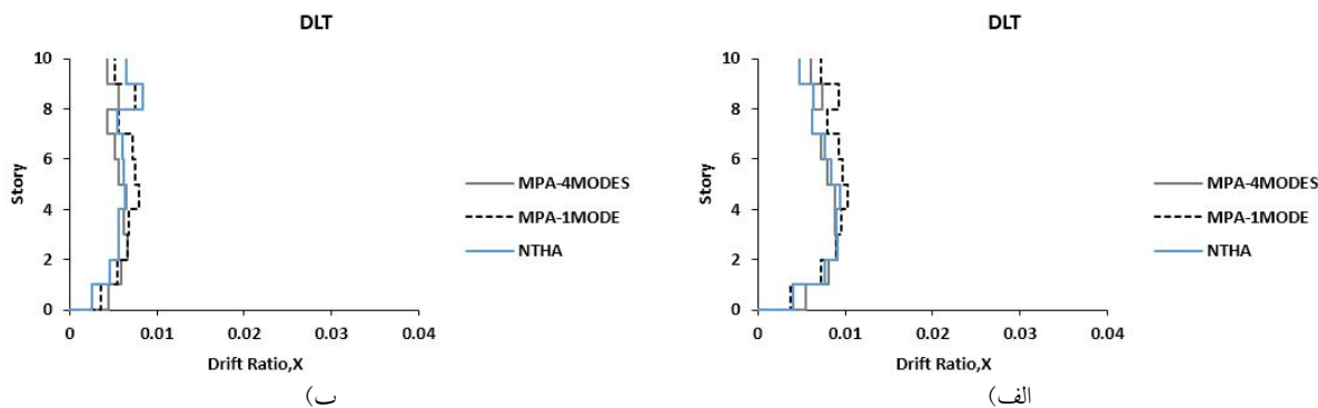
شکل ۱۲- پوش بیشینه دریفت در راستای X تحت رکورد مقیاس شده DLT: (الف) سازه Bundled Tube و (ب) سازه 3D FRAME (شکل ۳)
