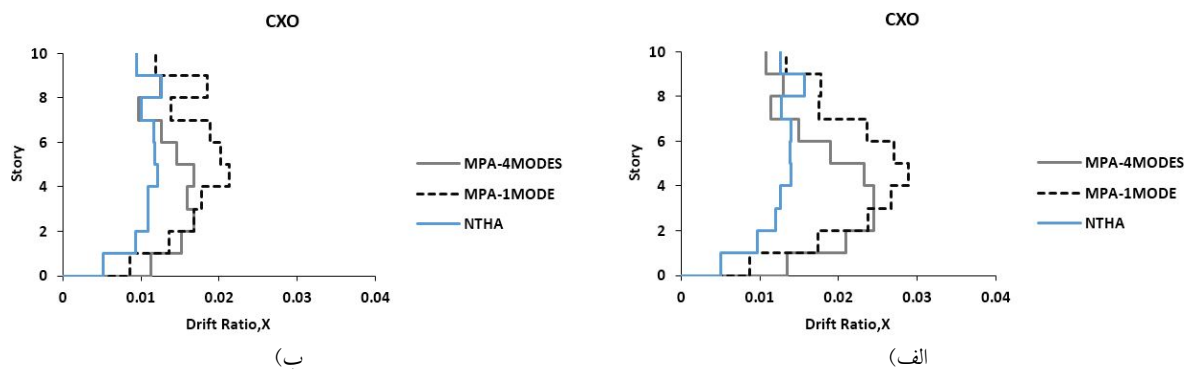
شکل ۱۱- پوش بیشینه دریفت در راستای X تحت رکورد مقیاس شده CXO: (الف) سازه Bundled Tube و (ب) سازه 3D FRAME (شکل ۳)
