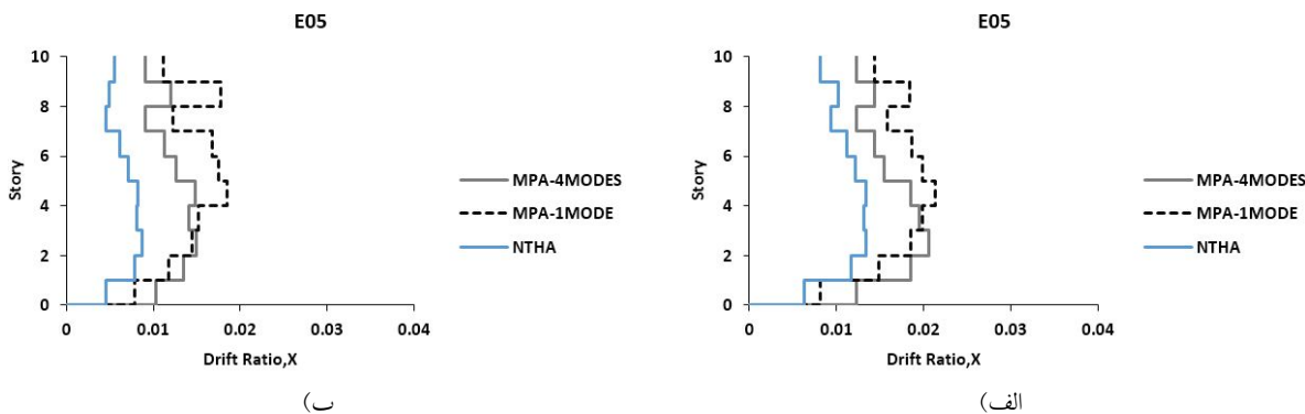
شکل ۱۳- پوش بیشینه دریفت در راستای X تحت رکورد مقیاس شده E05: (الف) سازه Bundled Tube و (ب) سازه 3D FRAME (شکل ۳)
