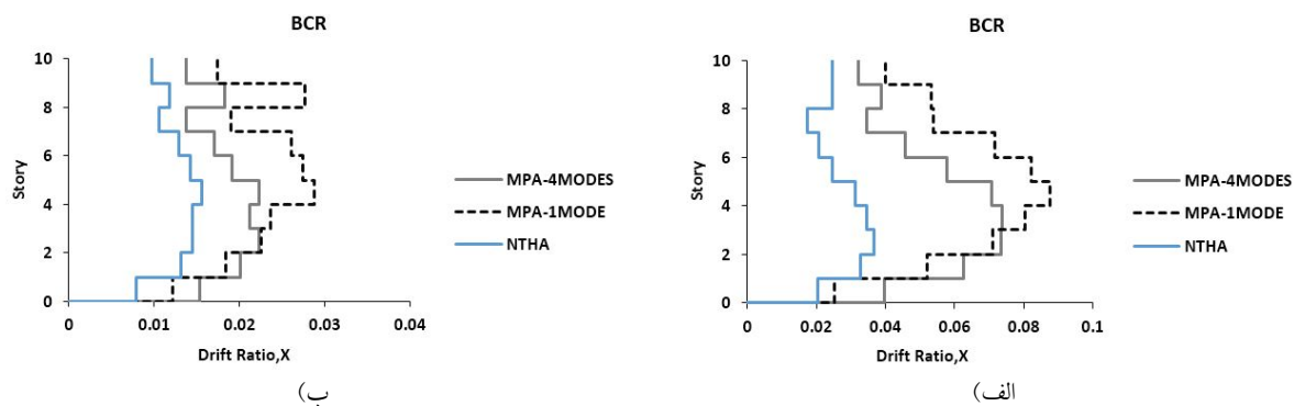
شکل ۱۰- پوش بیشینه دریفت در راستای X تحت رکورد مقیاس شده BCR: (الف) سازه Bundled Tube و (ب) سازه 3D FRAME (شکل ۳)
