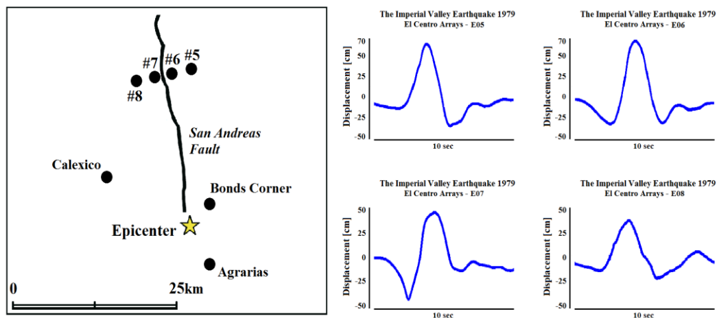
شکل ۱- حوزه لرزه خیز دره امپریال در زلزله ۱۹۷۹ کالیفرنیا و نمایش پالس‌های بردارانه و پیوسته تغییر مکان متناظر با مولفه TR رکورد ایستگاه‌های E05، E06، E07 و E08
