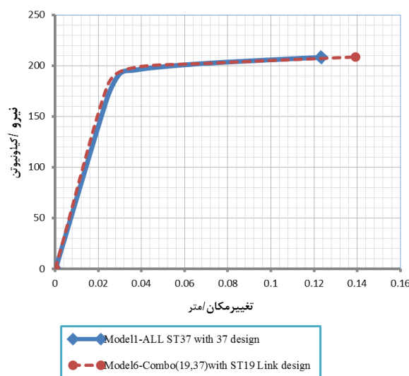
شکل (۱۱): مقایسه منحنی‌های پوش مدل‌های ۱ و ۶
