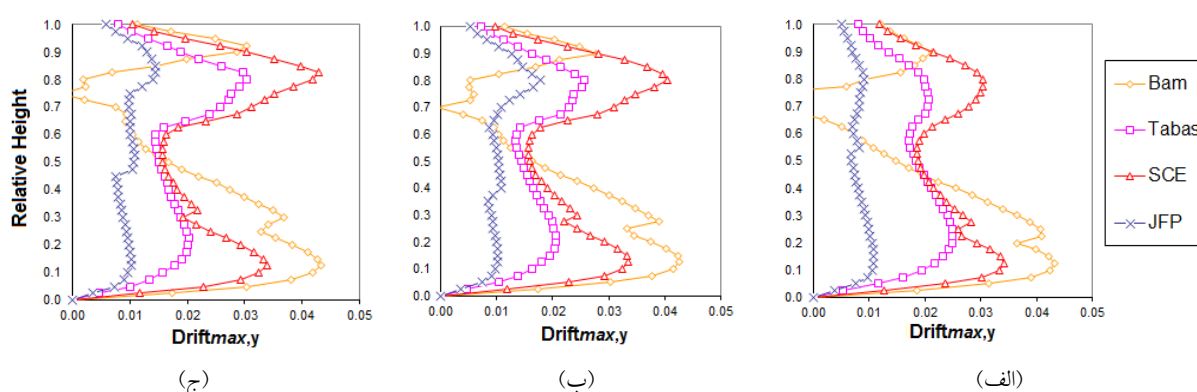
شکل ۱۶- پوش ماکزیمم دررفت طبقات در سازه‌های مطالعاتی ۴۰ طبقه: (الف) مدولاسیون یکنواخت، (ب) مدولاسیون ۵ طبقه‌ای و (ج) مدولاسیون ۴ طبقه‌ای
