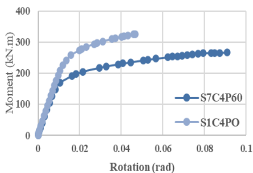
شکل ۲۰- منحنی لنگر - دوران نمونه‌های S7C4P60 و S1C4P0
