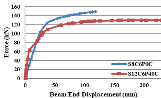
شکل ۲۲- منحنی بار - تغییر مکان S8C6P0 و S12C6P40
