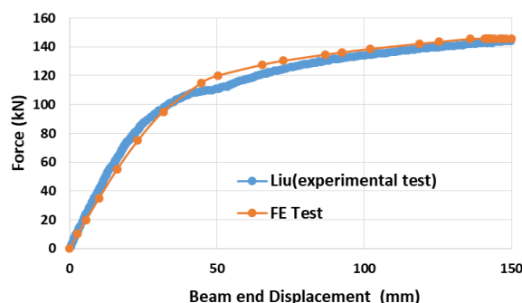
شکل ۹- مقایسه‌ی منحنی بار- تغییر مکان اتصال لئو و همکاران با مدل اجزای محدود پژوهش کنونی برای راستی‌آزمایی مدل‌سازی
