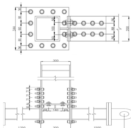
شکل ۸- نمایی از جزئیات هندسی اتصال پژوهش Liu و همکارانش [۱۷]
