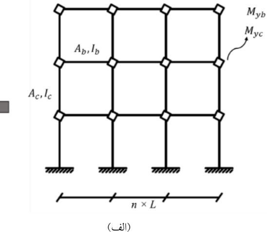
شکل ۸- (الف) مدل با جزئیات و (ب) قاب جایگزین
