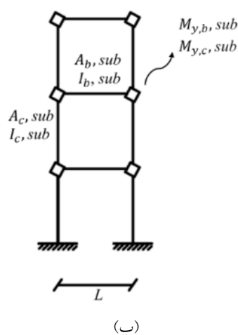
شکل ۸- (الف) مدل با جزئیات و (ب) قاب جایگزین
