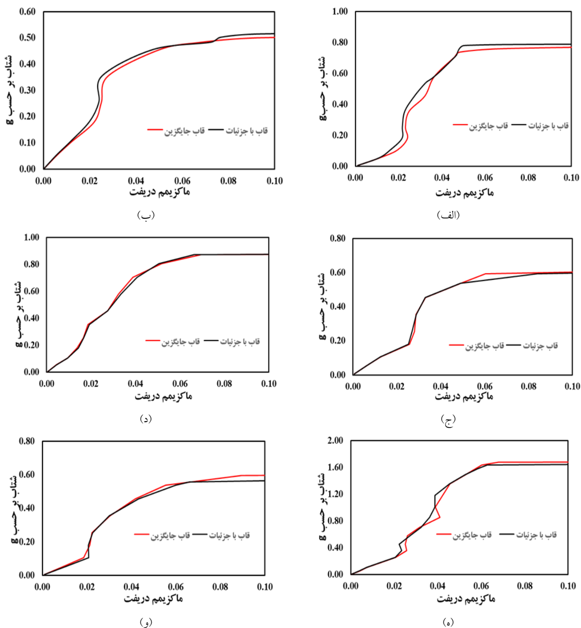
شکل ۱۰- نمودار منحنی‌های IDA: (الف) مدل ۸ طبقه (رکورد Northridge ایستگاه Mulhol)، (ب) مدل ۸ طبقه (رکورد Landers ایستگاه Yermo_Fire)، (ج) مدل ۱۲ طبقه (رکورد Hector mine ایستگاه Hector)، (د) مدل ۱۲ طبقه (رکورد Chi-Chi ایستگاه Chy101)، (و) مدل ۲۰ طبقه (رکورد Kobe ایستگاه Shin Osaka)، (ه) مدل ۲۰ طبقه (رکورد Imeprial valley ایستگاه EL cenntro)
