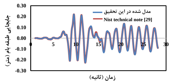
شکل ۷- تطابق نمودار جابجایی بر حسب زمان حاصل از مدل سازی در این تحقیق و گزارش برای رکورد kocaali ایستگاه Duzce180 [۲۹]
