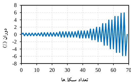
شکل ۷- تاریخیچه بارگذاری چرخه‌ای
