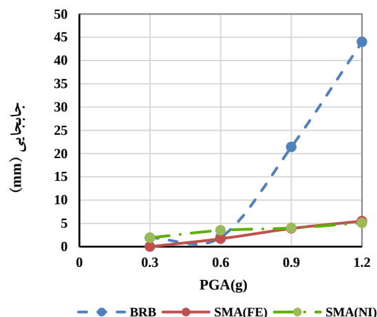
شکل ۲۵- مقایسه جابجایی مانده سیستم‌های سازه‌ای مختلف
