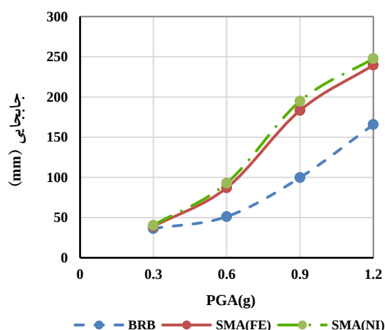
شکل ۲۴- مقایسه جابجایی حداکثر سیستم‌های سازه‌ای مختلف
