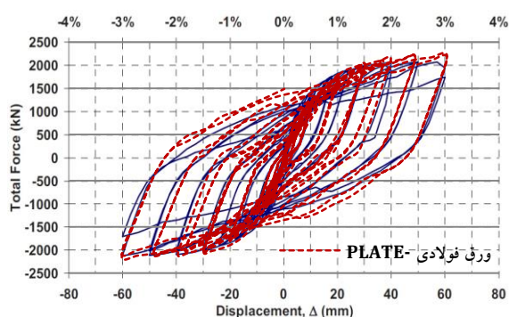
شکل ۵- رفتار هیستریزس نمونه آزمایشگاهی Ronny Purba و مقایسه مدل مذکور با مدل المان محدود قاب با ورق در آنالیز با نرم‌افزار ABAQUS [۹]
