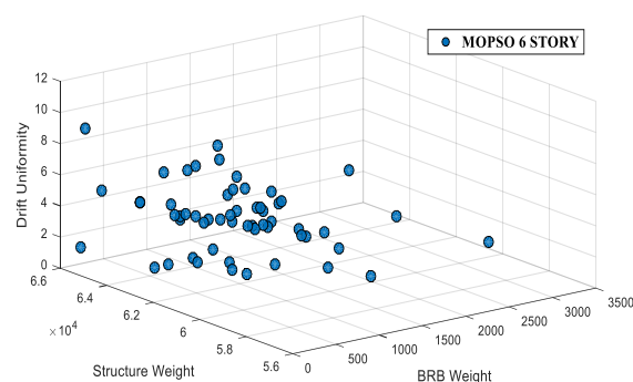
شکل ۷- نتایج الگوریتم بهینه‌سازی MOPSO برای سازه ۶ طبقه
