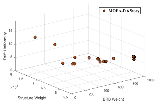
شکل ۹- نتایج الگوریتم بهینه‌سازی MOEA_D برای سازه ۶ طبقه
