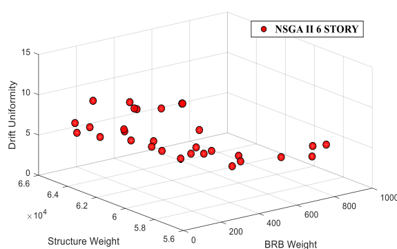
شکل ۸- نتایج الگوریتم بهینه‌سازی NSGA II برای سازه ۶ طبقه
