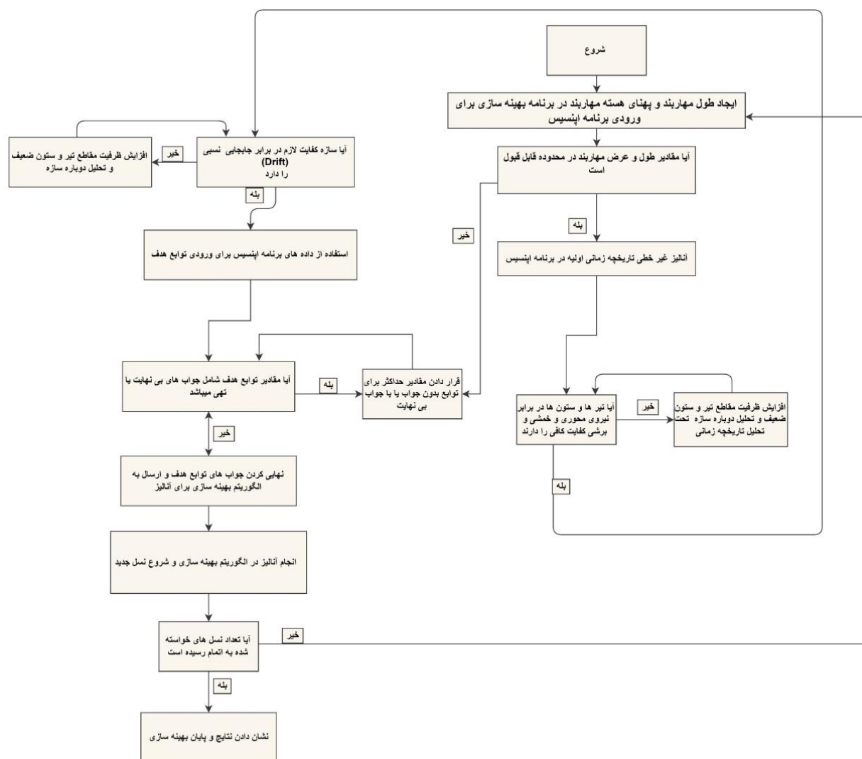
شکل ۶- مراحل مختلف به دست آوردن توابع هدف و تأثیر بعضی از قیود در برنامه OpenSees
