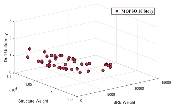
شکل ۱۳- نتایج بهینه‌سازی الگوریتم MOPSO برای سازه ۱۰ طبقه
