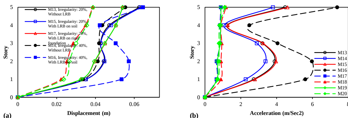
شکل ۱۷- نمودارهای مقایسه‌ای بیشینه پاسخ سازه ۵ طبقه دارای نامنظمی ۲۰٪ و ۴۰٪ برای حالت‌های M13، M14، M15، M16 و M17، (a) جابه‌جایی-زمان، (b) شتاب-زمان
