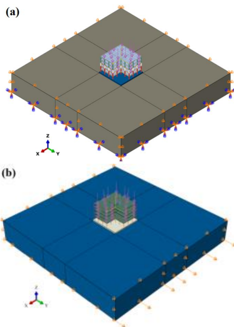
شکل ۵- شرایط بارگذاری و شرایط مرزی اعمال شده بر روی یک سازه نمونه، (a) بارگذاری استاتیکی، (b) بارگذاری دینامیکی غیرخطی
