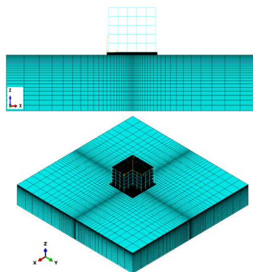
شکل ۶- نماهای دوبعدی و سه بعدی اجزای مختلف مدل های شبیه سازی شده در ABAQUS
