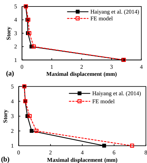
شکل ۷- پاسخ حداکثر جابه جایی طبقات در مقایسه با مدل آزمایشگاهی [۱۹] در حالت های (a) سازه روی پی خاک و (b) سازه روی پی صلب
