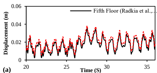
شکل ۸- (a) پاسخ جابه‌جایی-زمان و (b) نمودار پاسخ شتاب-زمان برای طبقه آخر سازه مدل‌سازی شده در مقایسه با مدل عددی [۲۶]
