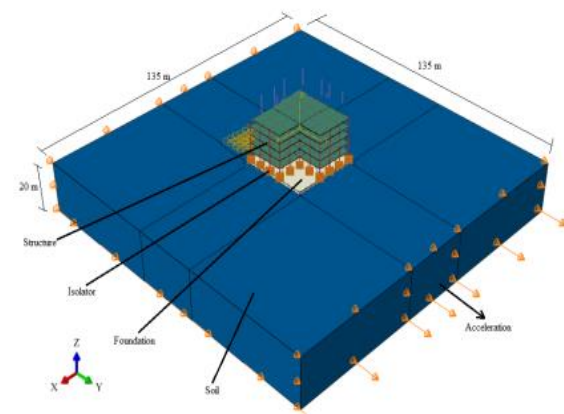
شکل ۲- نمای سه بعدی یک نمونه از مدل‌های سازه‌ای شبیه‌سازی شده در نرم‌افزار ABAQUS (سازه ۵ طبقه با نام‌نظمی ۰/۴۰٪)
