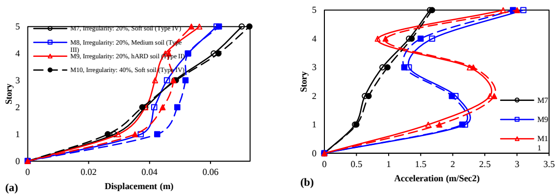
شکل ۱۶- نمودارهای مقایسه‌ای پیشینه پاسخ سازه‌های ۵ طبقه دارای نامنظمی ۲۰٪ و ۴۰٪ قرارگرفته بر روی خاک‌های نرم، متوسط و سخت، (a) جابه‌جایی-زمان، (b) شتاب-زمان
