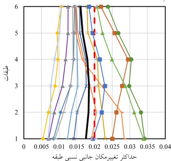
شکل ۸- حداکثر تغییر مکان جانبی نسبی طبقات مدل ۶ طبقه
