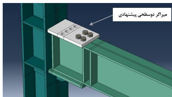
شکل ۱- میراگر دوسطحی پیشنهادی
