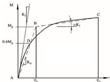
شکل ۲۷- ترسیم نمودار backbone و دوخطی معادل
