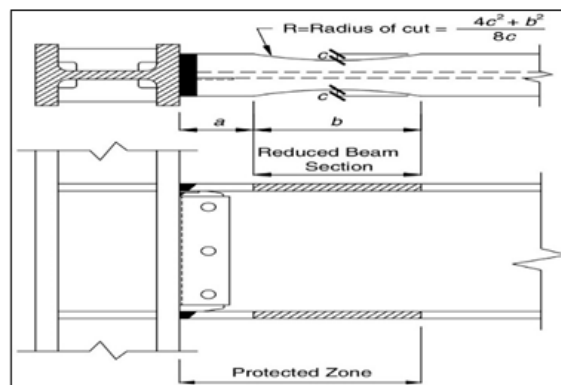
شکل ۲- برش شعاعی در اتصال با مقطع کاهش‌یافته [۹]
