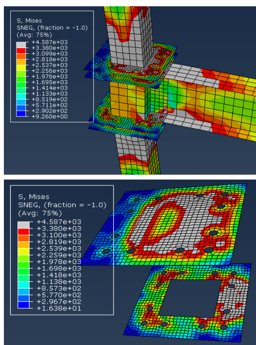
شکل ۱۰- کانتور تنش فون میسز در اتصال CBT18
