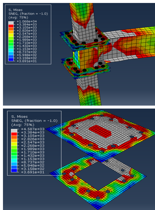
شکل ۸- کانتور تنش فون میسز در اتصال CBT15
