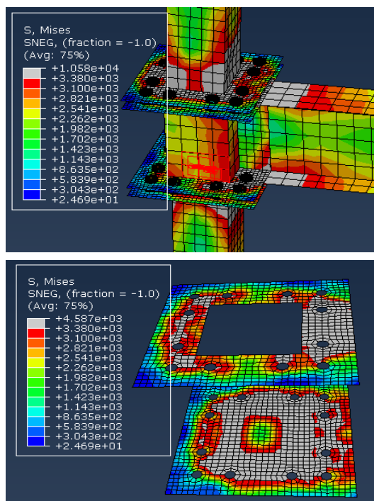
شکل ۶- کانور تنش فون میسیز در اتصال Ct12
