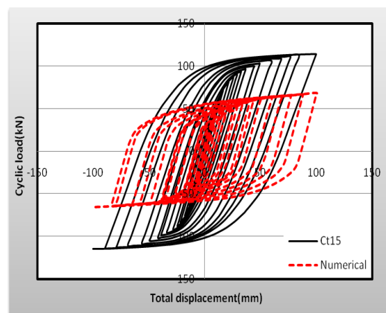
شکل ۹- منحنی بار-تغییر مکان در اتصال CBT15 و نمونه عددی
