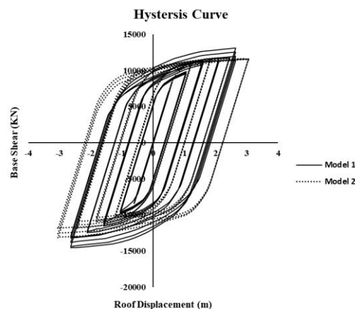
شکل ۸- مقایسه منحنی هیستریزیس دو مدل حاصل از تحلیل
