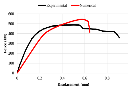
شکل ۱۰- نمودار نیرو-جابجایی مدل‌سازی عددی و آزمایشگاهی رن و همکاران [۳۰]
