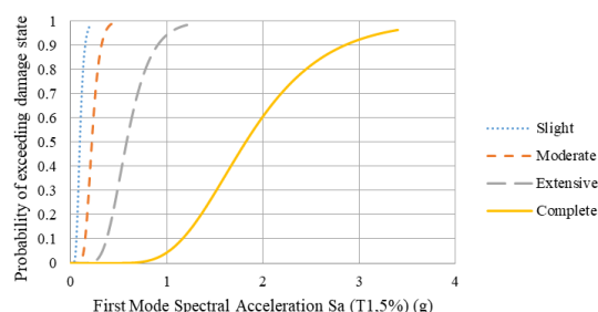
شکل ۱۴- نمودار منحنی شکنندگی قاب PT-2
