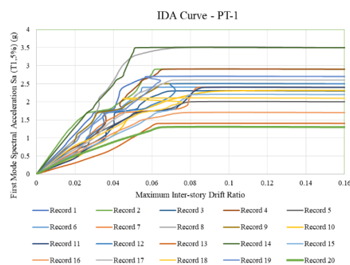
شکل ۹- منحنی تحلیل دینامیکی افزایشی مدل PT-1
