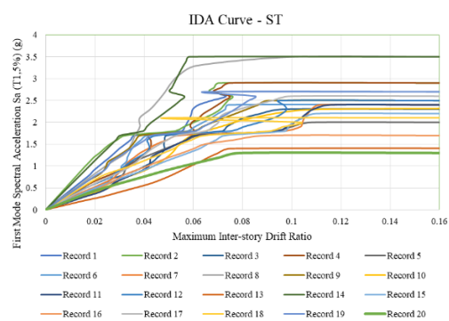
شکل ۱۰- منحنی تحلیل دینامیکی افزایشی مدل ST
