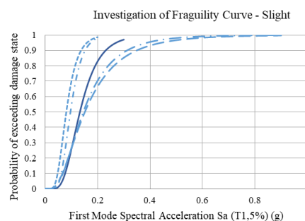
شکل ۱۷- منحنی شکنندگی مدل‌های تحقیق برای سطح عملکرد جزئی
