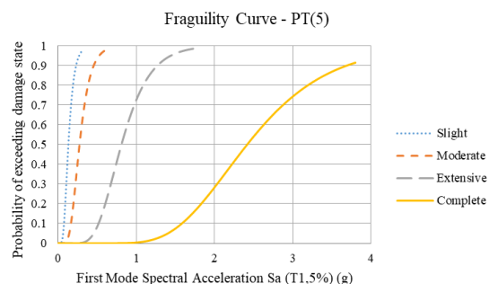
شکل ۱۱- نمودار منحنی شکنندگی قاب PT-5
