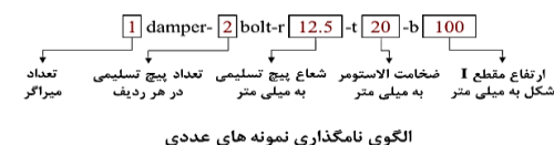
شکل ۲- مشخصات هندسی میراگر مورد بررسی (واحد mm)
