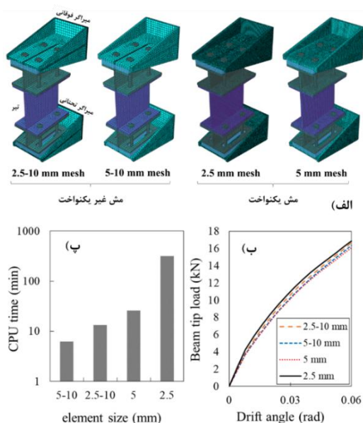
شکل ۱۰- تعیین اندازه مش در ناحیه میراگر؛ الف) نمونه مش‌بندی، ب) تغییرات نمودار نیرو-جابجایی، پ) تغییرات زمان تحلیل
