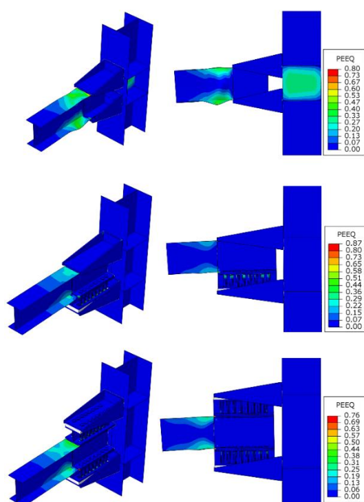
شکل ۲۳- توزیع کرنش پلاستیک تجمعی در اتصال فاقد میراگر، اتصال دارای میراگر با پیکربندی ۲ و قطر پیچ ۲۱/۵ میلی‌متر (دررفت ۶٪)
