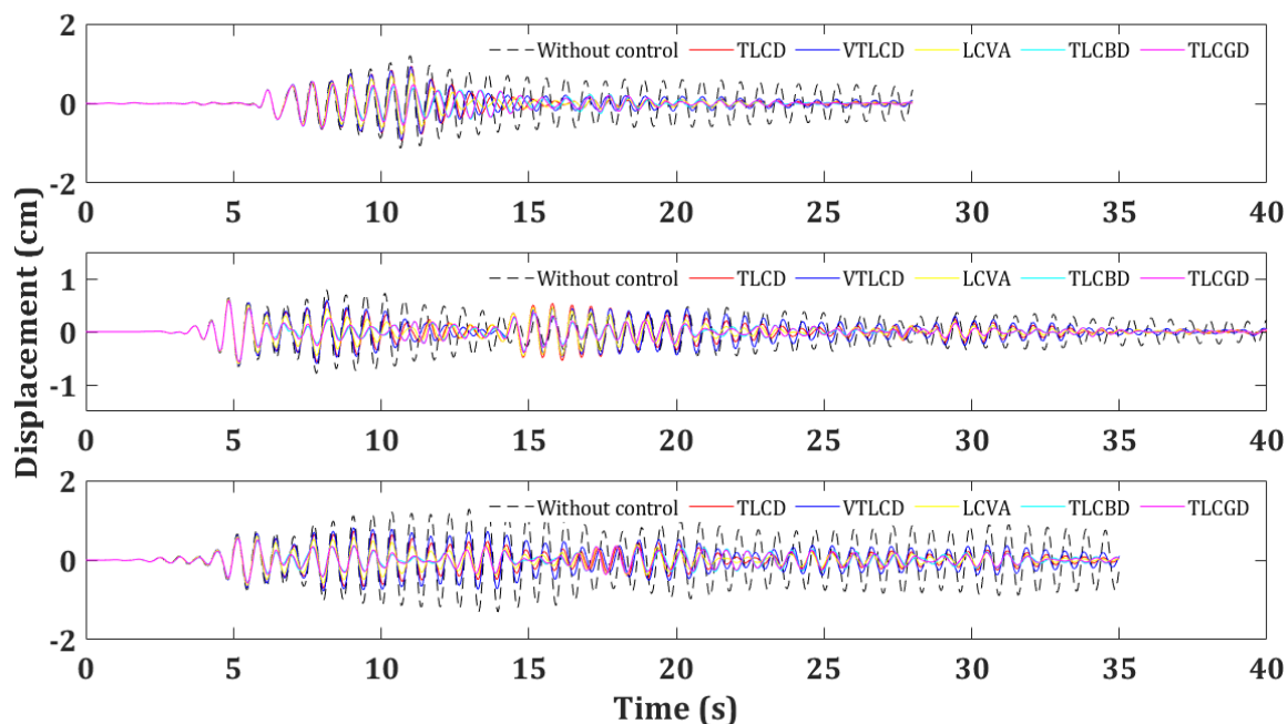
شکل ۶- تاریخچه زمانی پاسخ جابه‌جایی سقف سازه برای زلزله: الف) کوبه، ب) ال‌سترو و ج) تفت
