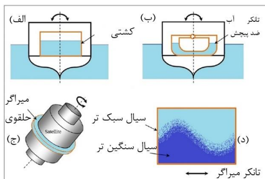
شکل ۱- توسعه اولیه میراگر TLD: (الف) تانکر آب ضدپیمش در کشتی، (ب) تانکر ضدپیمش U شکل در کشتی، (ج) میراگر حلقوی در کشتی و (د) میراگر سیالی با دو سیال مخلوط نشدنی. (فلش‌های دو جهته بیانگر جهت تحریک برای کنترل توسط وسیله میراگر می‌باشد). [۳۰]
