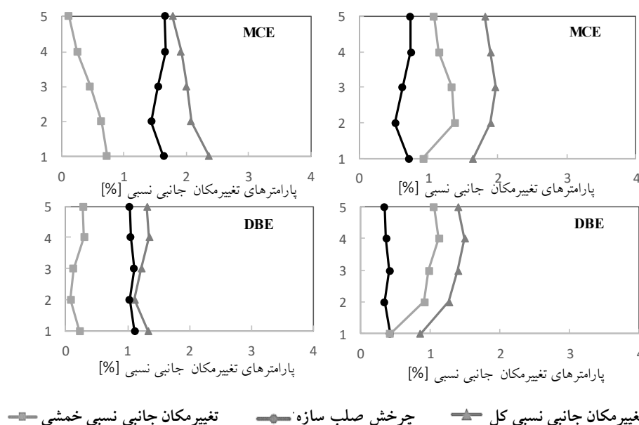
شکل ۱۷- مؤلفه‌های تغییرمکانی سازه در قاب‌های فولادی دارای پای ثابت و گهواره‌ای
