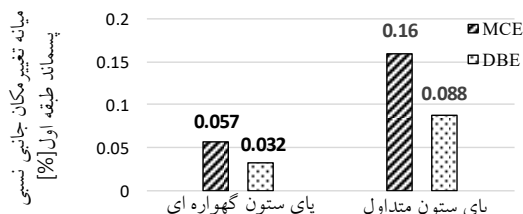
شکل ۱۶- میانه تغییر مکان جانبی نسبی پسماند طبقه اول
