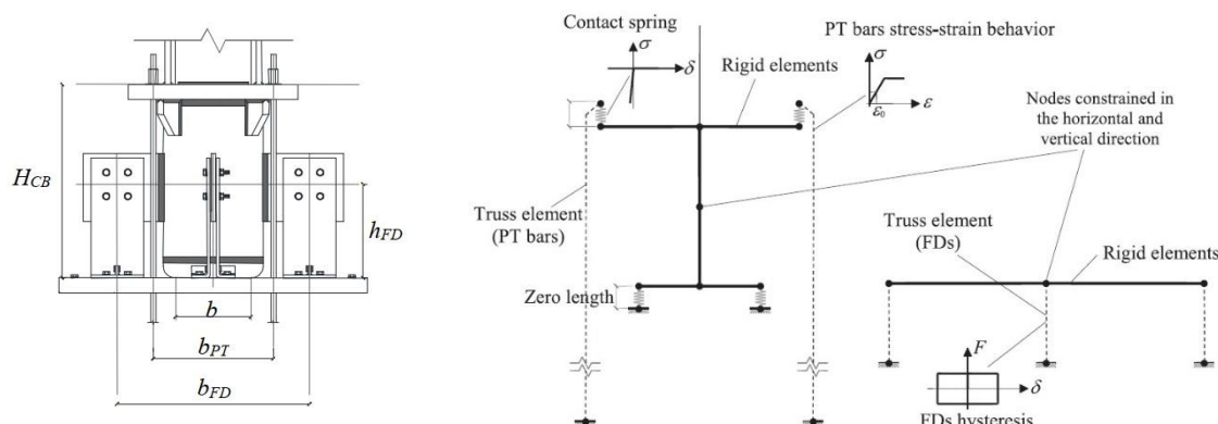
شکل ۷- پارامترهای هندسی پایه ستون گهواره‌ای [۱۰]
