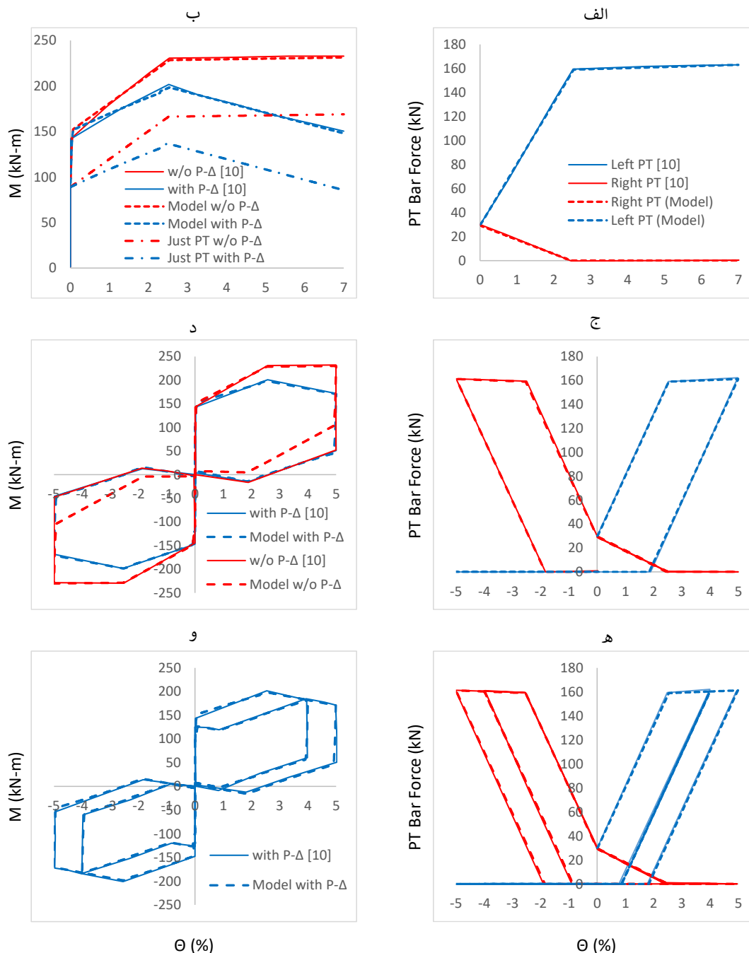
شکل ۹- نمونه‌ای از فرآیند صحت‌سنجی مدل‌های عددی در زیربخش پای ستون بر اساس نمودارهای نیروی کششی-دوران پایه و لنگر-دوران پایه تحت تأثیر: الف) و ب) جابه‌جایی‌های یک‌گانه، ج) و د) یک چرخه ۵ درصدی، ه) و و) دو چرخه ۴ و ۵ درصدی
