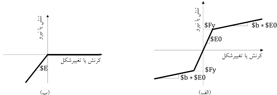
شکل ۴- منحنی‌های رفتاری مورد استفاده در مدل عددی [۳۱]: الف) مصالح فولاد ۰۱، ب) مصالح ارتجاعی بدون کشش
