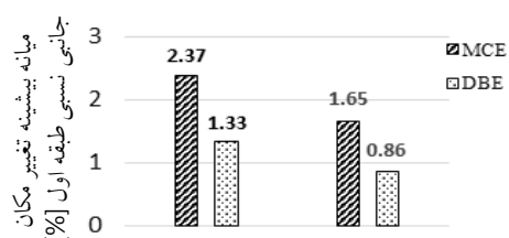
شکل ۱۴- مقادیر میانه بیشینه تغییر مکان جانبی نسبی طبقه اول پای ستون متداول پای ستون گهواره‌ای
