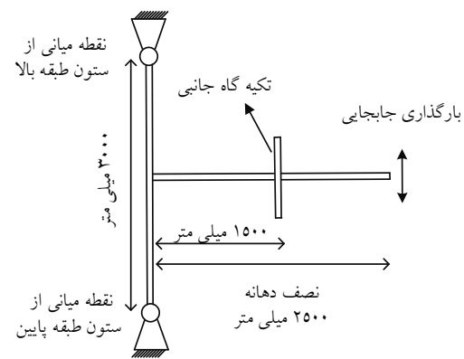
شکل ۵- شرایط مرزی نمونه مرجع
