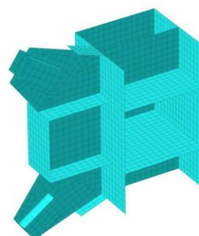
شکل ۲۰- نحوه تعبیه سخت کننده عمودی در محل اتصال ورق های گاست به ستون
