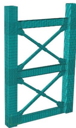
شکل ۱۸- نمای کلی از قاب تحلیل شده در نرم افزار آباکوس
