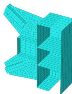
شکل ۱۹- نحوه استیفرگذاری افقی در محل اتصال ورق های گاست به ستون
