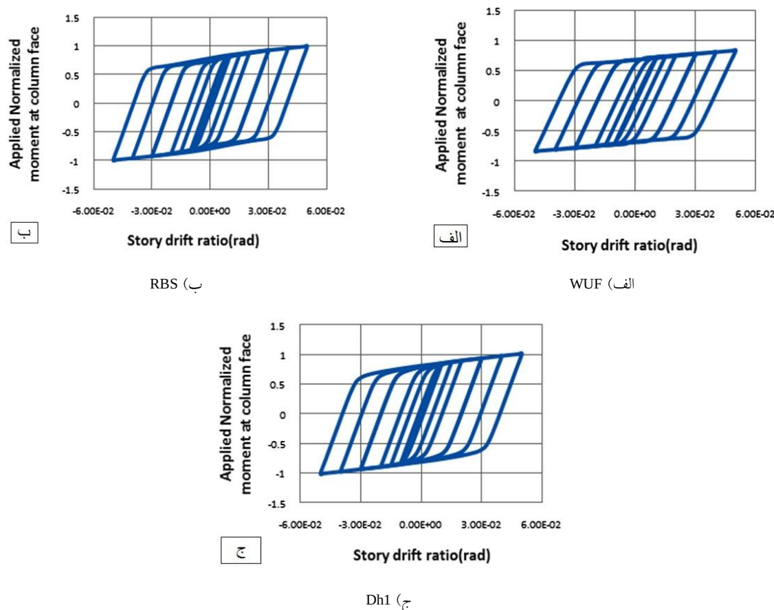
شکل ۸- نمودار هیستریزیس مدل‌های تحلیلی برای نسبت مقاومتی V_{pzm}/V_y = 0.7
