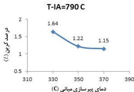
شکل (۹): درصد وزنی کربن در آستنیت باقیمانده در نمونه‌های D، B و E
