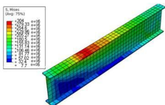
شکل ۱۲- توزیع تنش میسر روی تیر مدل SP5 در آخرین مرحله بارگذاری چرخه‌ای (Pa)
