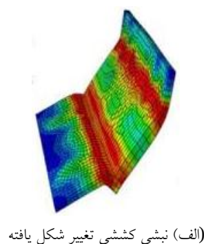
شکل ۱۴- نحوه تغییر شکل اتصال پس کشیده و ایجاد مفصل پلاستیک در نبشی های کششی و فشاری
