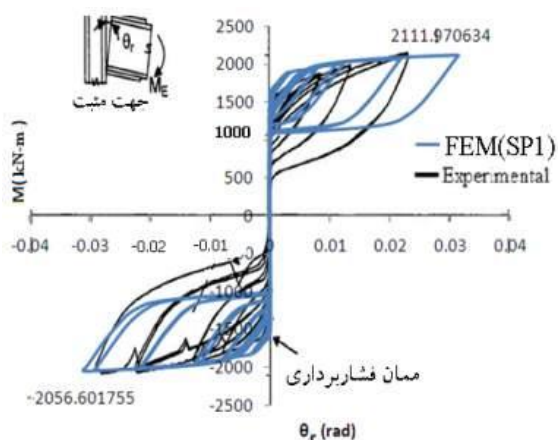
شکل ۹- مقایسه نمودار ممان خمشی- زاویه شکاف بدست آمده از تحلیل عددی و نتایج آزمایشگاهی مدل SP1
