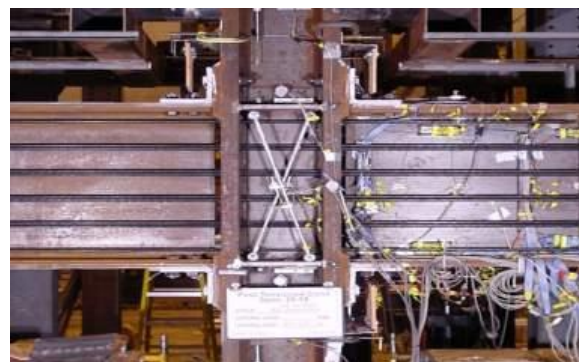
شکل ۲- نمونه آزمایشگاهی اتصالات فولادی پس کشیده همراه با نبشی‌های فوقانی و تحتانی [۳]
