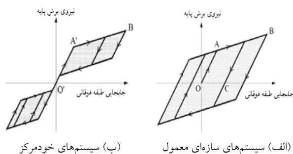
شکل ۱- نمودار هیستریزیس ایده آل نیرو-جابجایی [۴]
