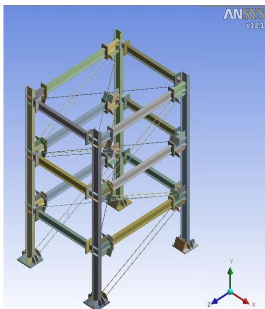
شکل ۲- مدل سازه در ANSYS Workbench
