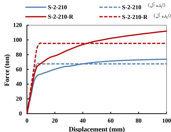
ج) ورق با تنش تسلیم ۲۱۰ MPa
