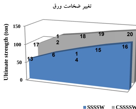
شکل ۸- تأثیر تغییرات ضخامت ورق بر مقاومت نهایی سیستم در حالت تقویت نشده (SSSSW) و تقویت شده با الیاف (CSSSSW)
