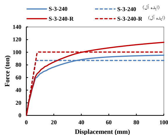
ج) ورق با ضخامت ۳ mm
