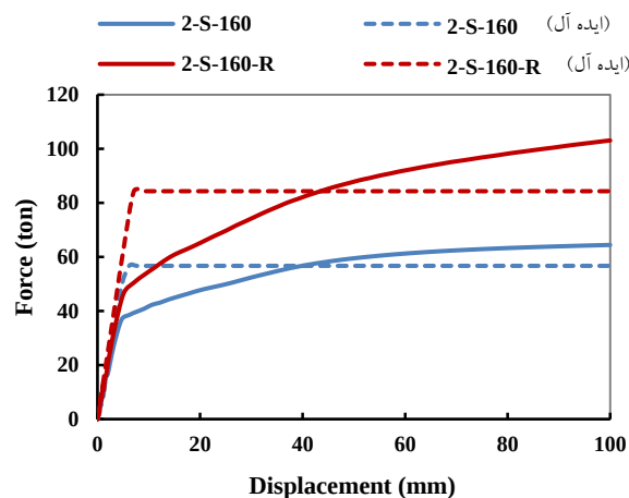
الف) ورق با تنش تسلیم ۱۶۰ MPa
