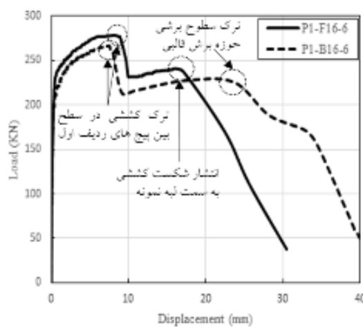
شکل ۷- منحنی های بار-جابجایی نمونه های P1-F16-6 و P1-B16-6
